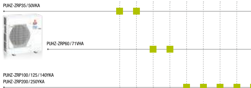
PUHZ-ZRP35/50VKA
