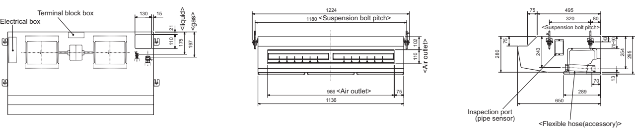
Urządzenia podstropowe ze stali nierdzewnej PCA-RP71HAQ
