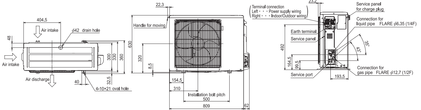
Urządzenia zewnętrzne Power Inverter, PUZ-ZM / PUHZ-ZRP35 / 50 VHA
