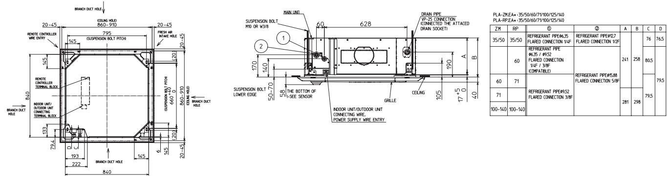
Urządzenia kasetonowe 4-stronne PLA-ZM / RP35-140 EA
